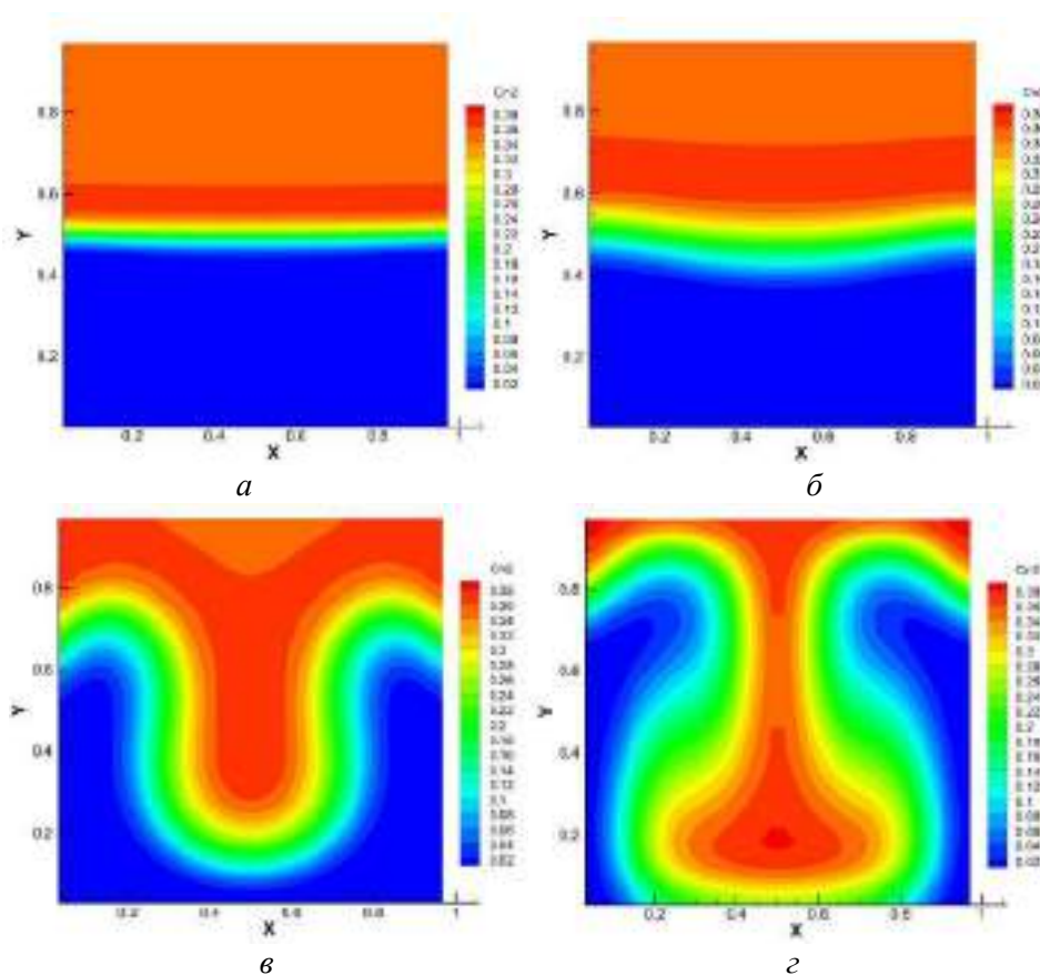
Рисунок 1. Динамика изменения концентрации фреона-12 по времени при p=0,5 МПа, T=298,0 К, L=165 \cdot 10^{-3} м, r=3 \cdot 10^{-3} м: а) t=4,6 с; б) t=8,78 с; в) t=18,8 с; з) t=20,7 с
