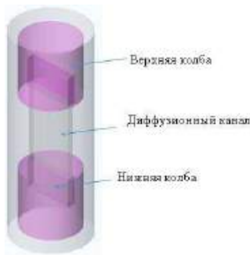
Рисунок 1. Виртуальная численная модель двухколбового аппарата
