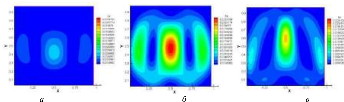
Рисунок 2. Распределение кинетической энергии для системы 0,65He+0,35R 12 -Ar при p=0.5 МПа, T = 298,0 К, L = 165 \cdot 10^{-3} м, r = 3 \cdot 10^{-3} м: а) t = 12,5 с; б) t = 18,8 с; в) t = 20,7 с
