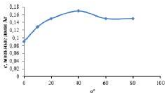
Рисунок 3. Зависимость концентрации Ag в ядре образовавшейся структуры от угла наклона диффузионного канала \alpha
