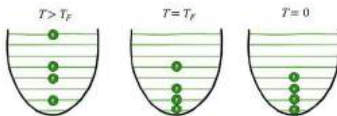
Сурет 3. Паули принципіне бағынатын бөлшектер үшін энергетикалық деңгейлер
