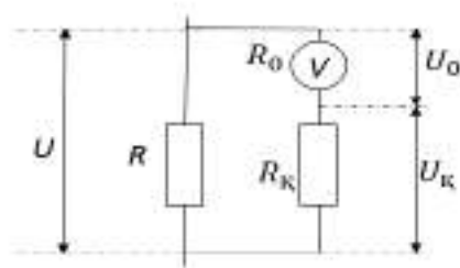
Сурет 2. Вольтметрдің өлшеу шегін кеңейту
