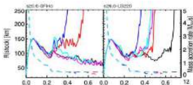
Сурет 4. Уақыттың жұлдыз радиусынан (сол жақта) және аккреция жылдамдығынан (оң жақта) тәуелділігі. Есептеулер нәтижелері мюондарды есепке алғанда – қара сызықпен, мюондарды есепке алмағанда – қызыл сызықпен белгіленген
